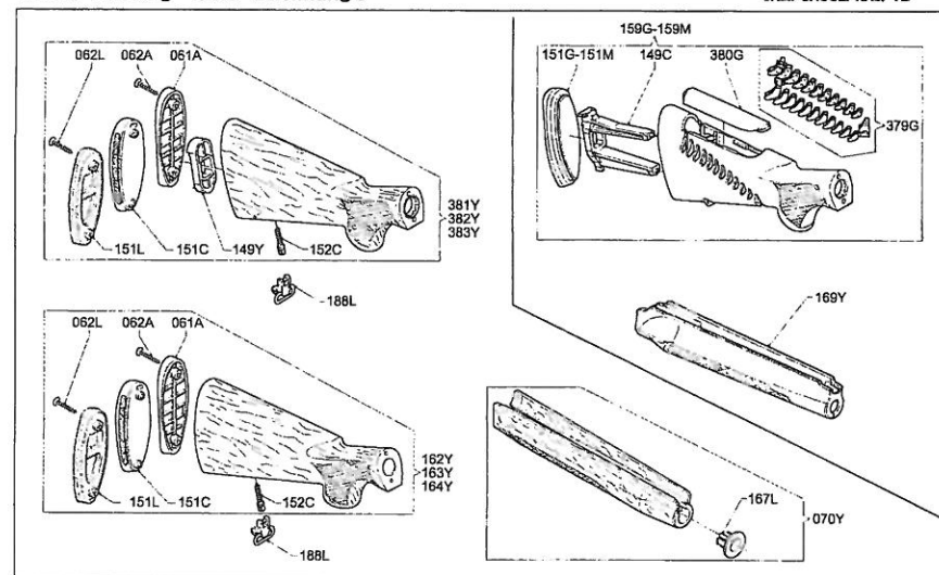
Tavola - Drawing - Table - Zeichnung 5
