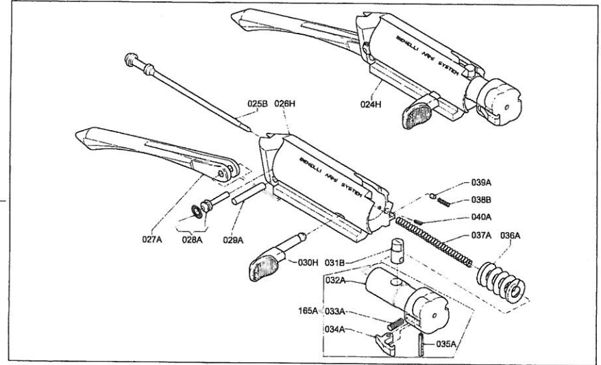
Tavola - Drawing - Table - Zeichnung 2
