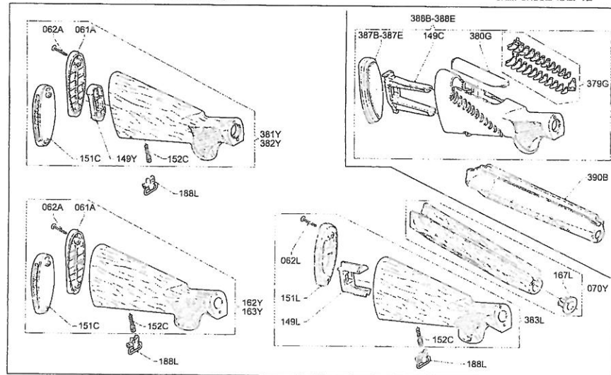
Tavola - Drawing - Table - Zeichnung 9
