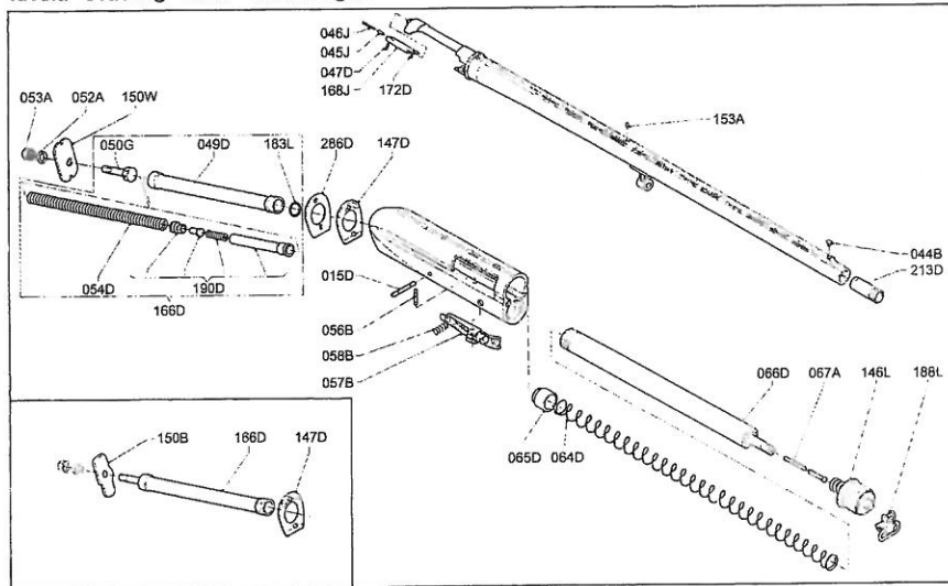
Tavola - Drawing - Table - Zeichnung 12
