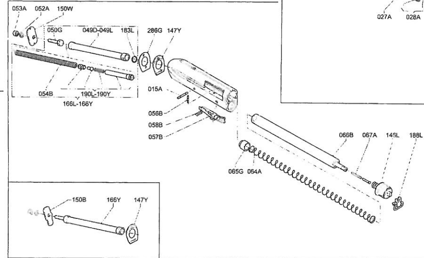
Tavola - Drawing - Table - Zeichnung 3
