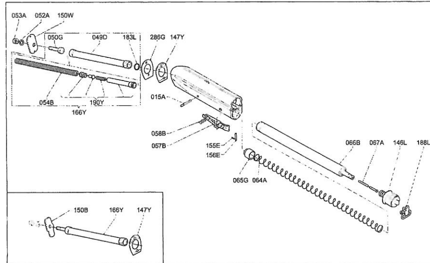
Tavola - Drawing - Table - Zeichnung 7
