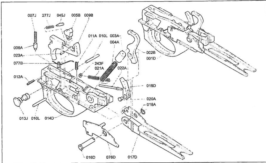
Tavola - Drawing - Table - Zeichnung 10
