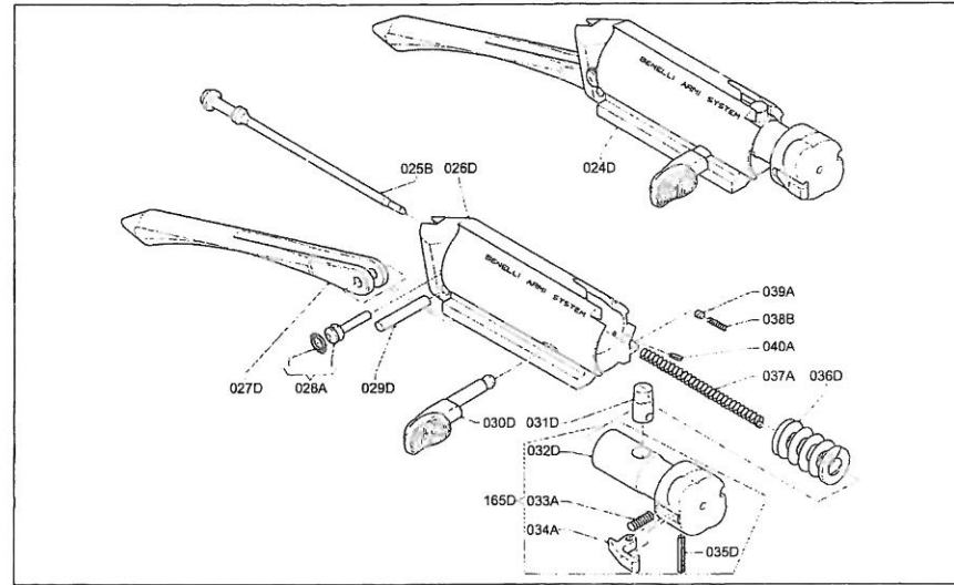
Tavola - Drawing - Table - Zeichnung 11
