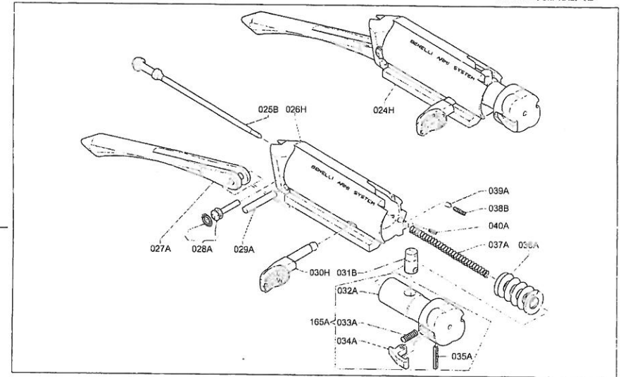
Tavola - Drawing - Table - Zeichnung 2
