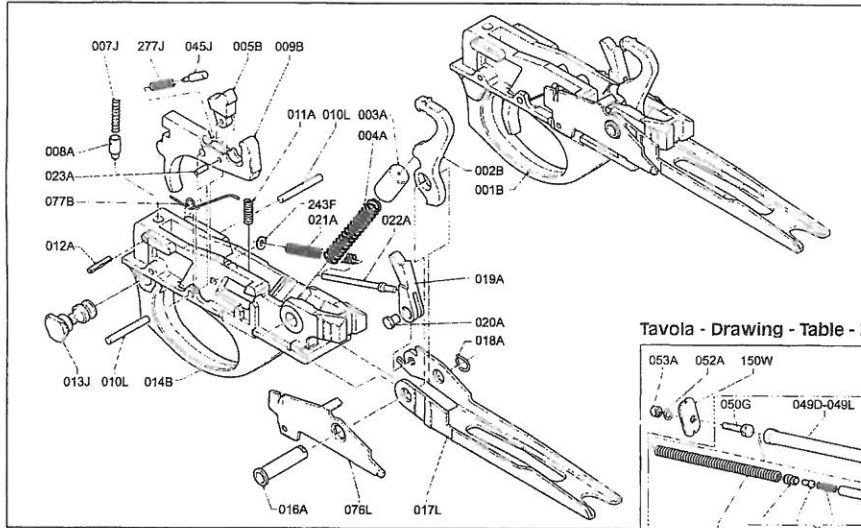
Tavola - Drawing - Table - Zeichnung 1
